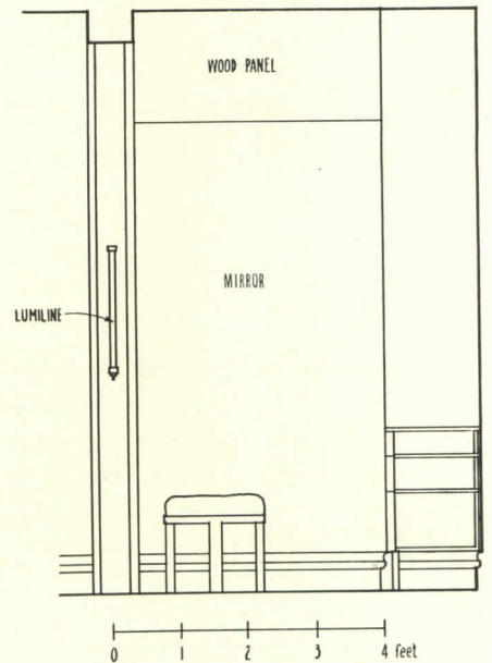
Elevation
