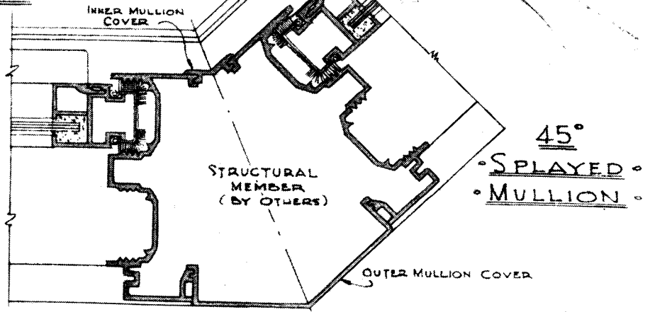
• JAMB SECTION •
