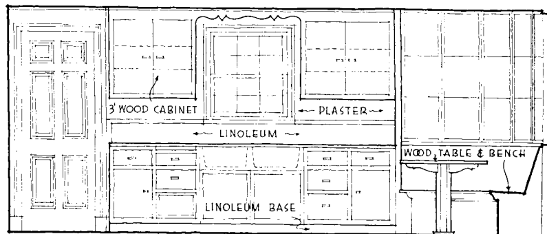
ELEVATION A
