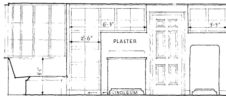
ELEVATION B
