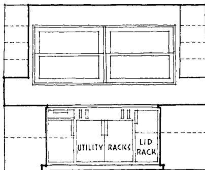
ELEVATION B
