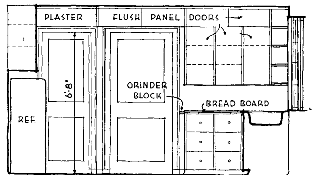
ELEVATION A
