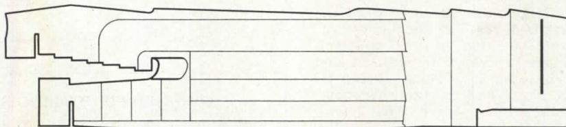
LONGITUDINAL SECTION
