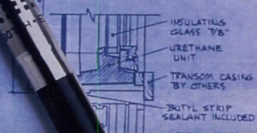
HEAD-JAMB (SIMILAR) SCALE 3"=10"
