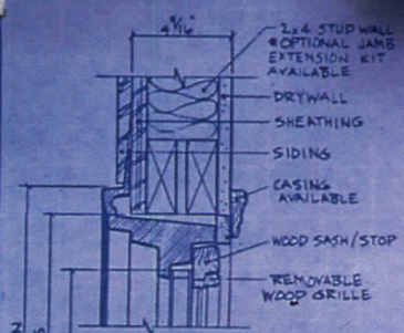
HEAD-JAMB (SIMILAR) SCALE 3"=10"
